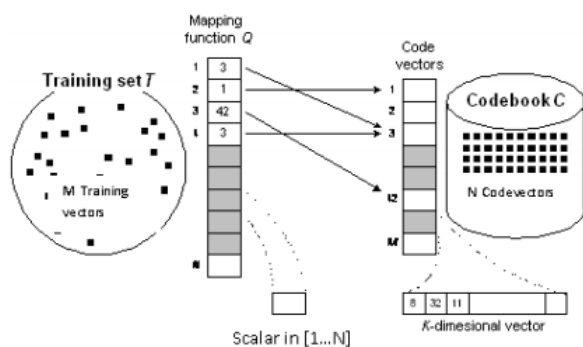
Fig4 : VQ Encoder [10]
