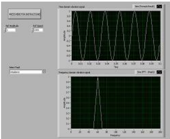
Fig. 6 Pure Imbalance
